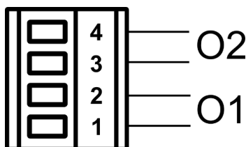
Obr. 5: Připojení výstupů
