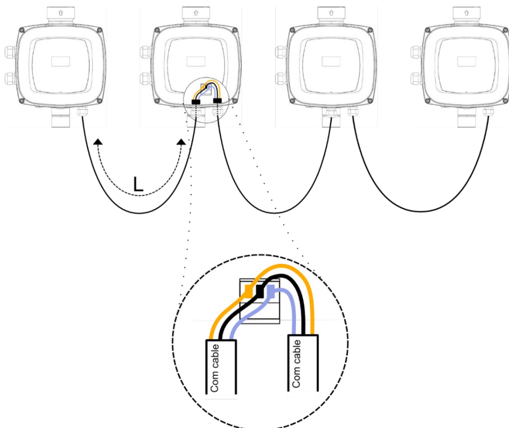
Obr. 6: Příklad připojení komunikace multi invertor se 4 zařízeními
