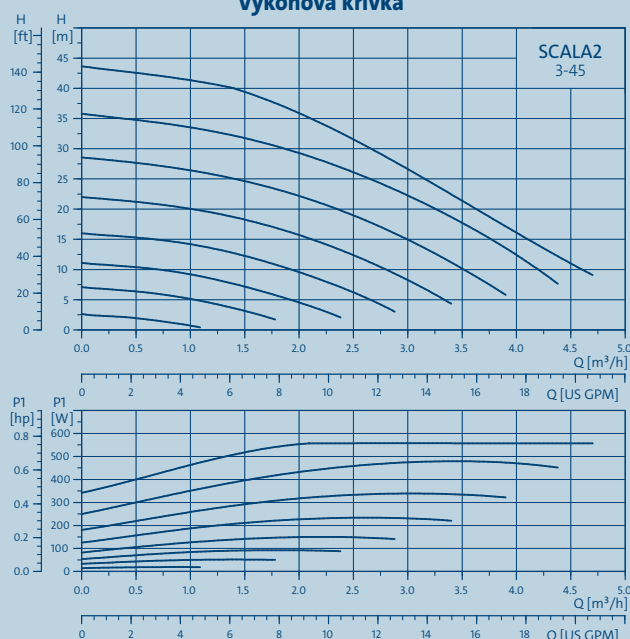
Výkonová křivka
