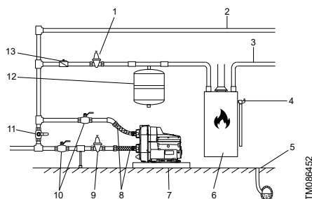
Příklad instalace
