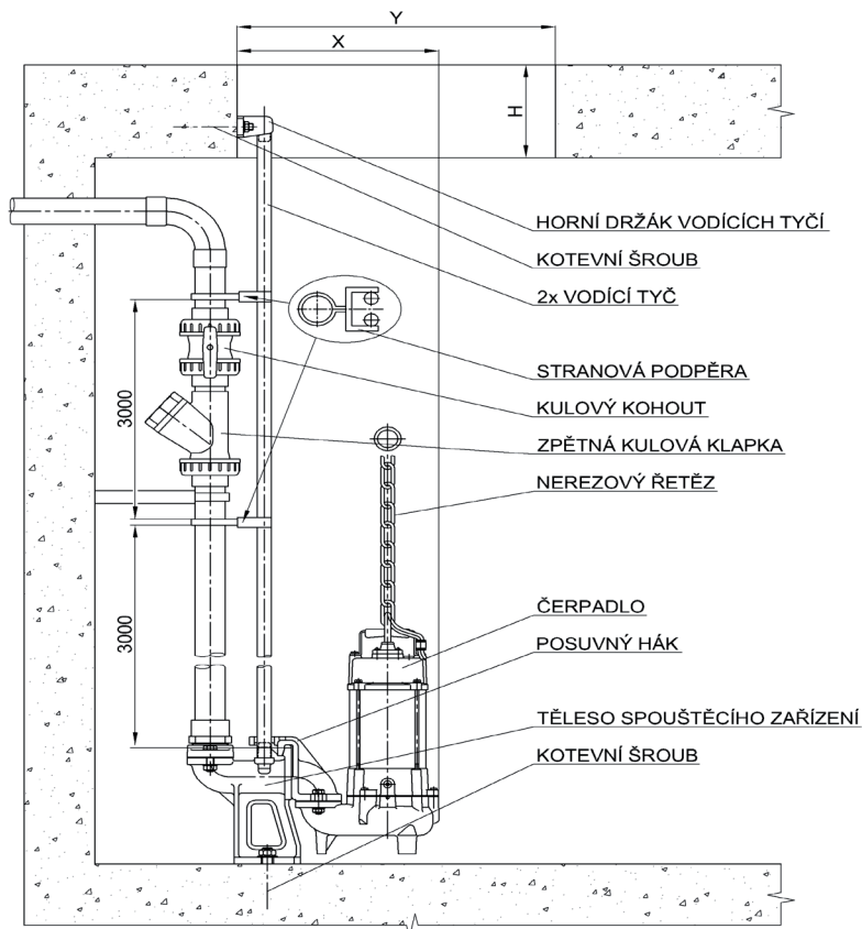
Obr. spouštěcího zařízení čerpadla
