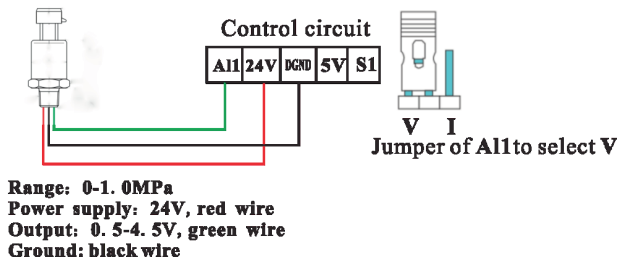
Obrázok 3.3 Senzor tlaku s napäťovou zpetnou väzbou
