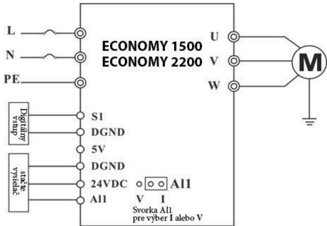
Obrázok 3.1 Elektrická schéma
