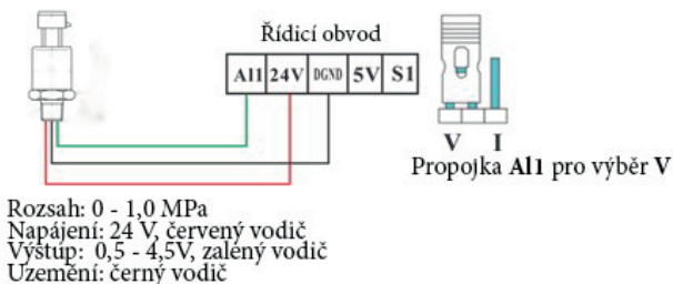
Obrázek 3.3 Senzor tlaku s napěťovou zpětnou vazbou
