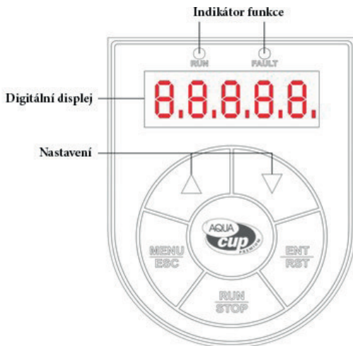
Obrázek 4.1 Schéma klávesnice
