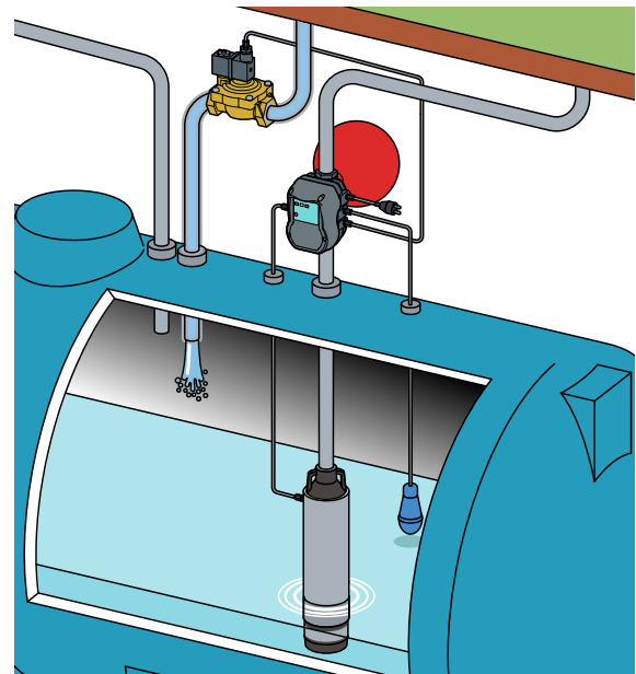
Čerpadlo mimo provoz Kontakty plováku rozepnuty Elektroventil otevřen - probíhá dopouštění
