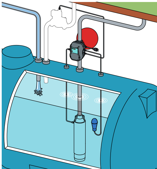
Čerpadlo v automatickém provozu Kontakty plováku sepnuty Elektroventil zavřen
