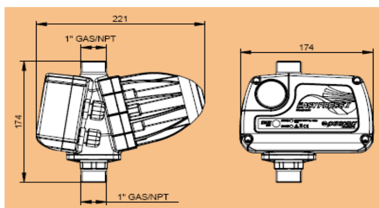
Rozměry [mm]
