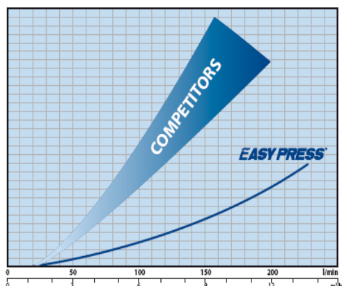
Hydraulické ztráty [m H 2 O]
