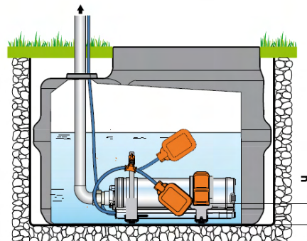
Horizontální instalace
