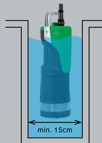
Rozměry vrtu/studny
