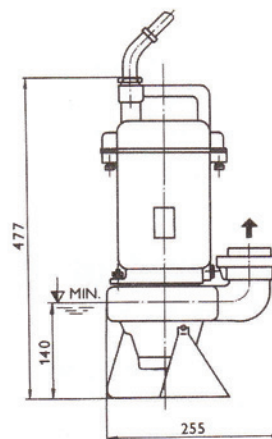
Trojfázové provedení
