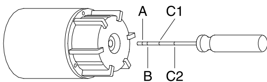
Obr. 5 Měření vzdálenosti spodní desky k membráně
