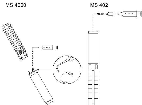
Obr. 2 Poloha motoru při plnění - MS 4000 a MS 402
