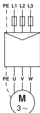
Obr. 14 Motory Grundfos - přímé spouštění
