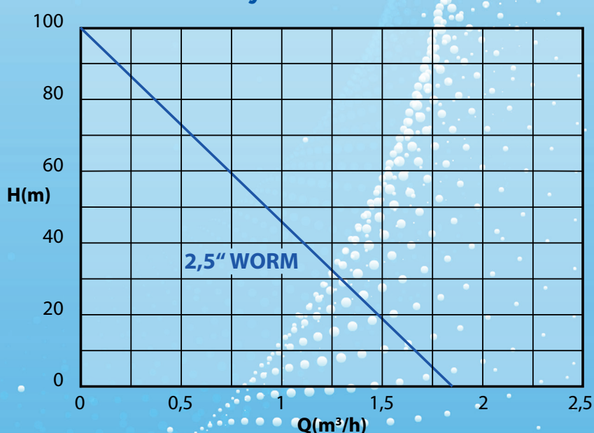
Výkonová křivka
