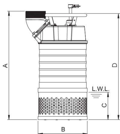
VERTIKÁLNÍ VÝTLAK
