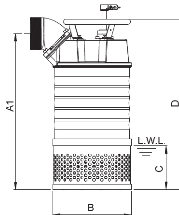
HORIZONTÁLNÍ VÝTLAK
