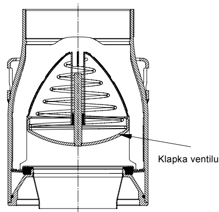
Obr. 5 Zpětný ventil
