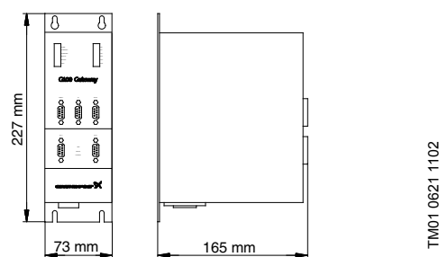
Obr. 24 Rozměrový náčrtek
