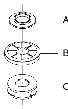
Obr. 7 Stavěcí kroužek (otočná a pevná část) a dělený kuželový element
