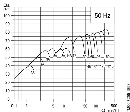
Obr. 1 Stupeň účinnosti čerpadla/motoru v závislosti na průtoku
